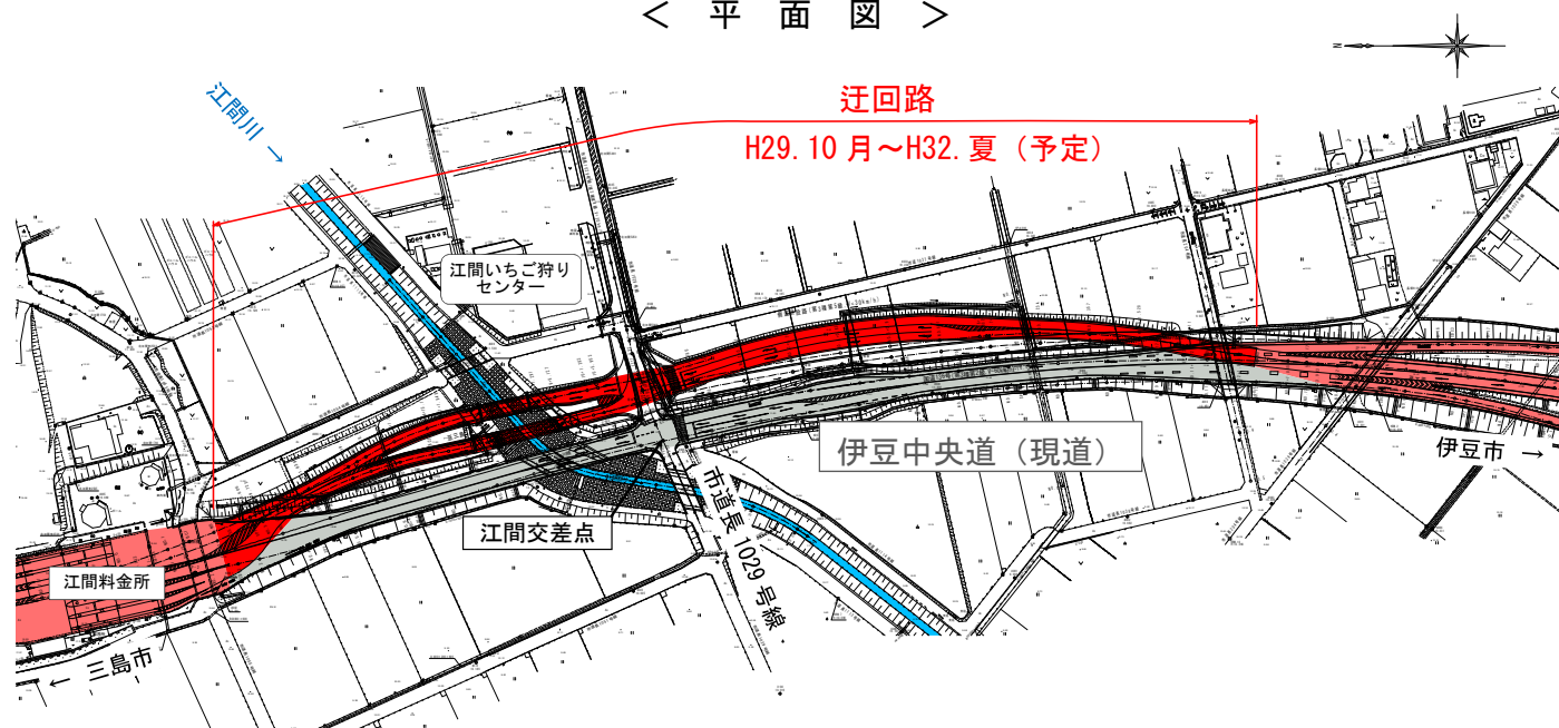
< 平面図 >
